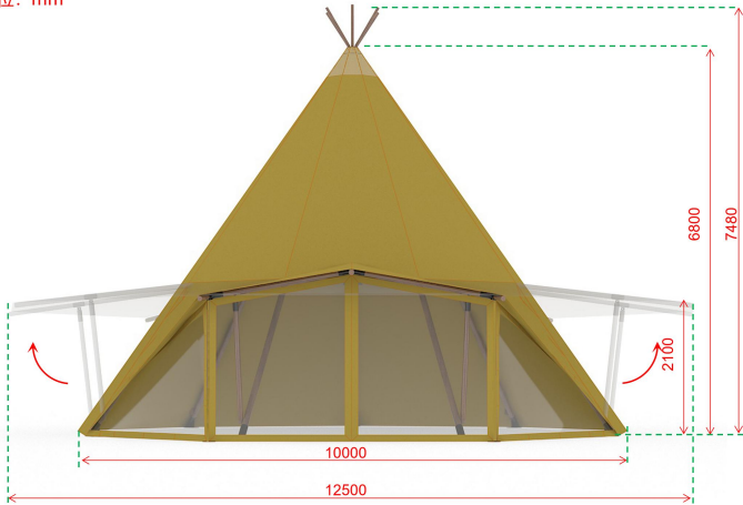
印第安餐厅帐尺寸图
