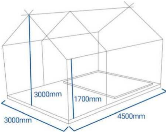
B-400 Tent dimensions
