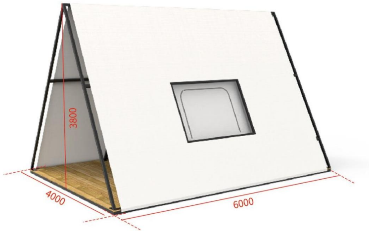
K -200 Tent Dimensions
